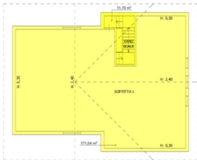
PIANTA PIANO TERZO Scala 1:100
